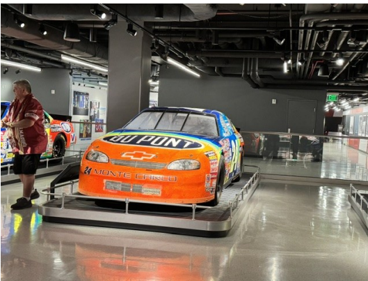
Monte Carlo
